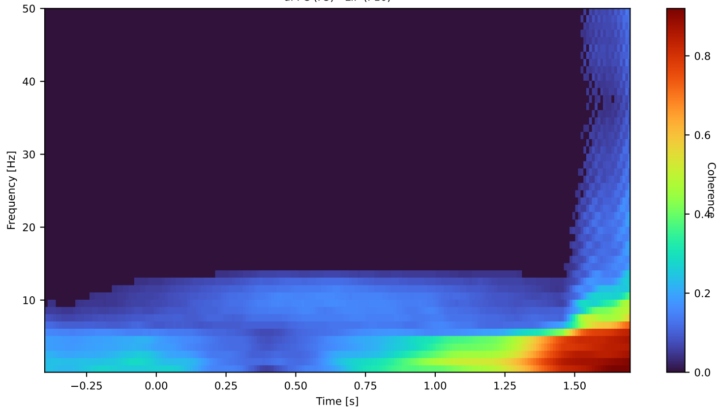
dPFC (F5) - LIP (P10)
